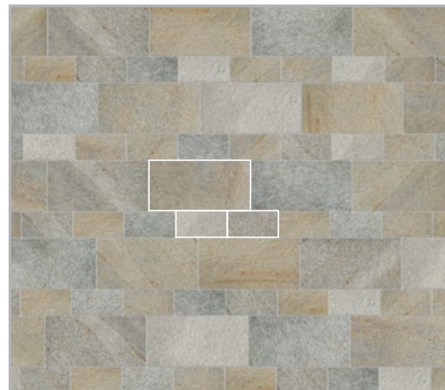
30x60 - (12"x24") 66,7% 15x30 (6"x12") 33,3%
